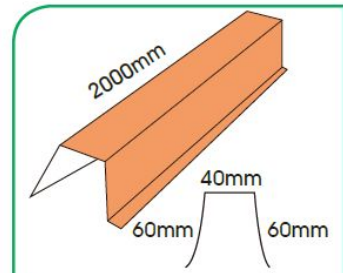
Square Rige Cap
